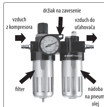
Obr. 10, popis jednotky na úpravu Extol® 8865105
