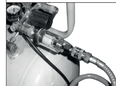
Abb. 8, Anschluss vom Filter (Abscheider) Extol® Craft 8865101
