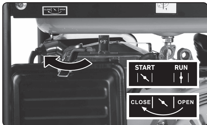
Obr. 16, přepnutí páčky sytiče do pozice „start“ nebo „close“ dle šítku
