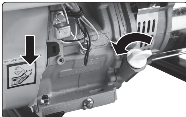
Abb. 9, Verschluss des Einfüllstutzens für Öl, Etikett mit dem richtigen Ölstand im Tank
