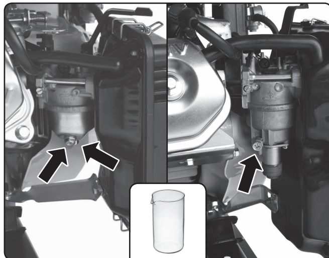
Odkalenie v prípade modelu 421000
